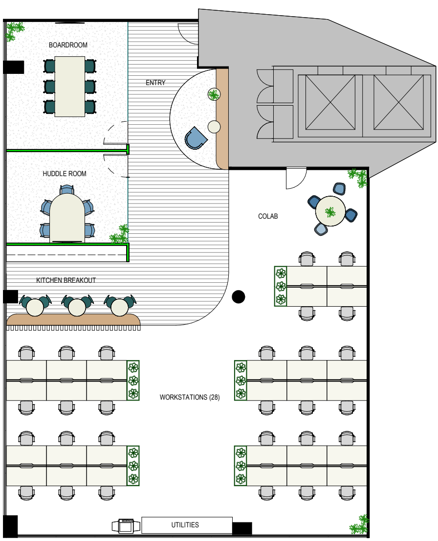
1 OPTION 1 1:100
